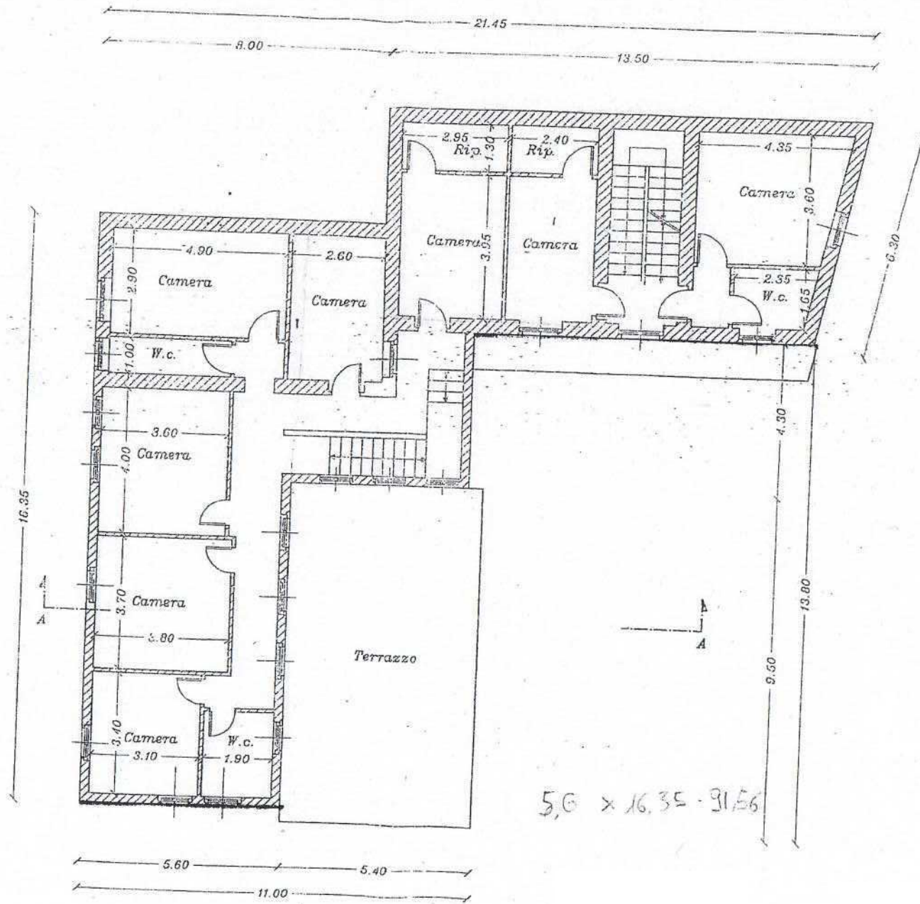
PIANTA PIANO SECONDO
